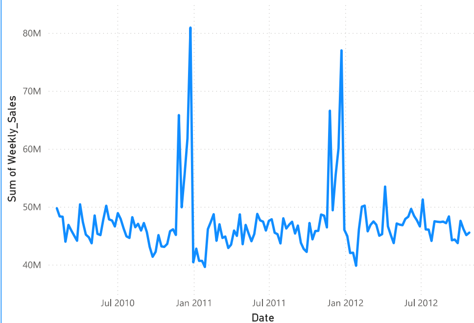
Actual Sales
